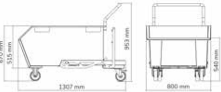
BENNA PORTAROTTAMI RIBALTABILE CAPACITÀ 300 L CON RUOTE PREDISPOSTA PER GRIGLIA E RUBINETTO
